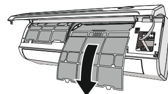
Защелки фильтра
